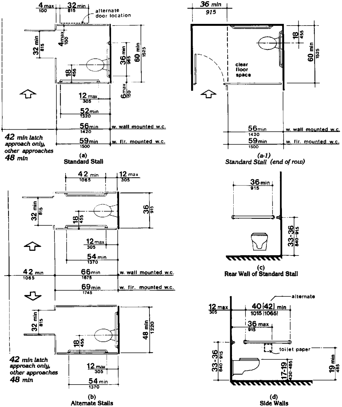
Fig. 30 Toilet Stalls
