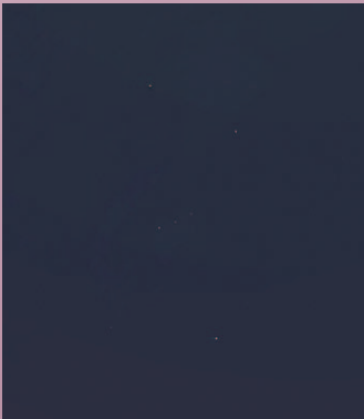
Magnitude 2
