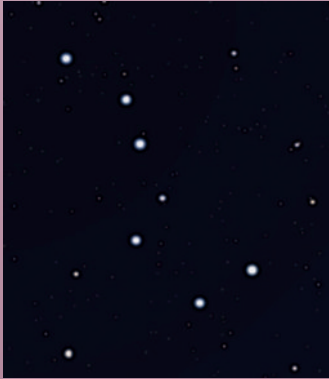
Magnitude 7
