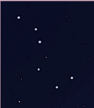
Magnitude 6
